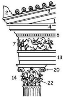
Onderdelen bouworde
